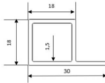
Профиль для полки из ЛДСП
