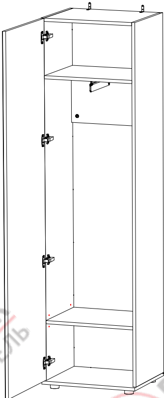
Левый шкаф
