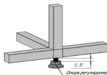
Опора регулируемая
